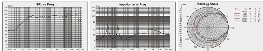
PS-80频响曲线
