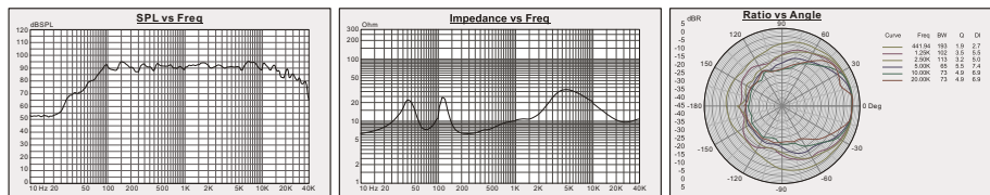
PS-60频响曲线
