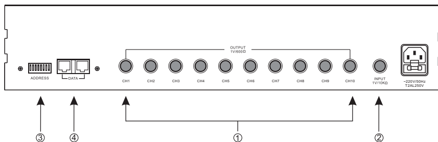
后面板
