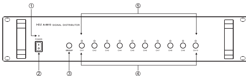
前面板
